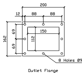
Outlet Flange
