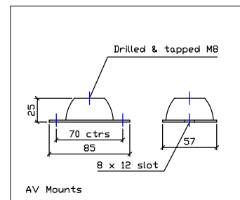
AV Mounts
